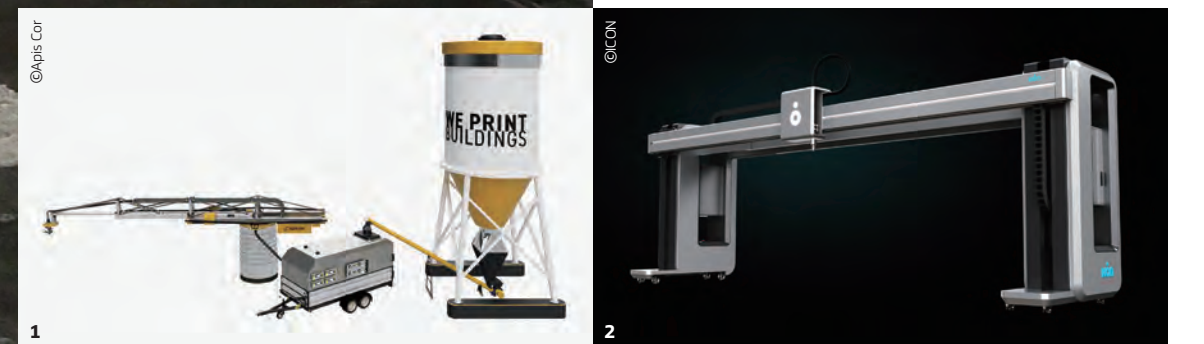
1, 2 아피스 코어의 건축용 3D 프린터는 로봇 팔 타입이고(왼쪽) 폭이 8.5m에 달하는 아이콘의 벌컨 II는 일반적인 3D 프린터를 크게 확대한 모습이다(오른쪽).
